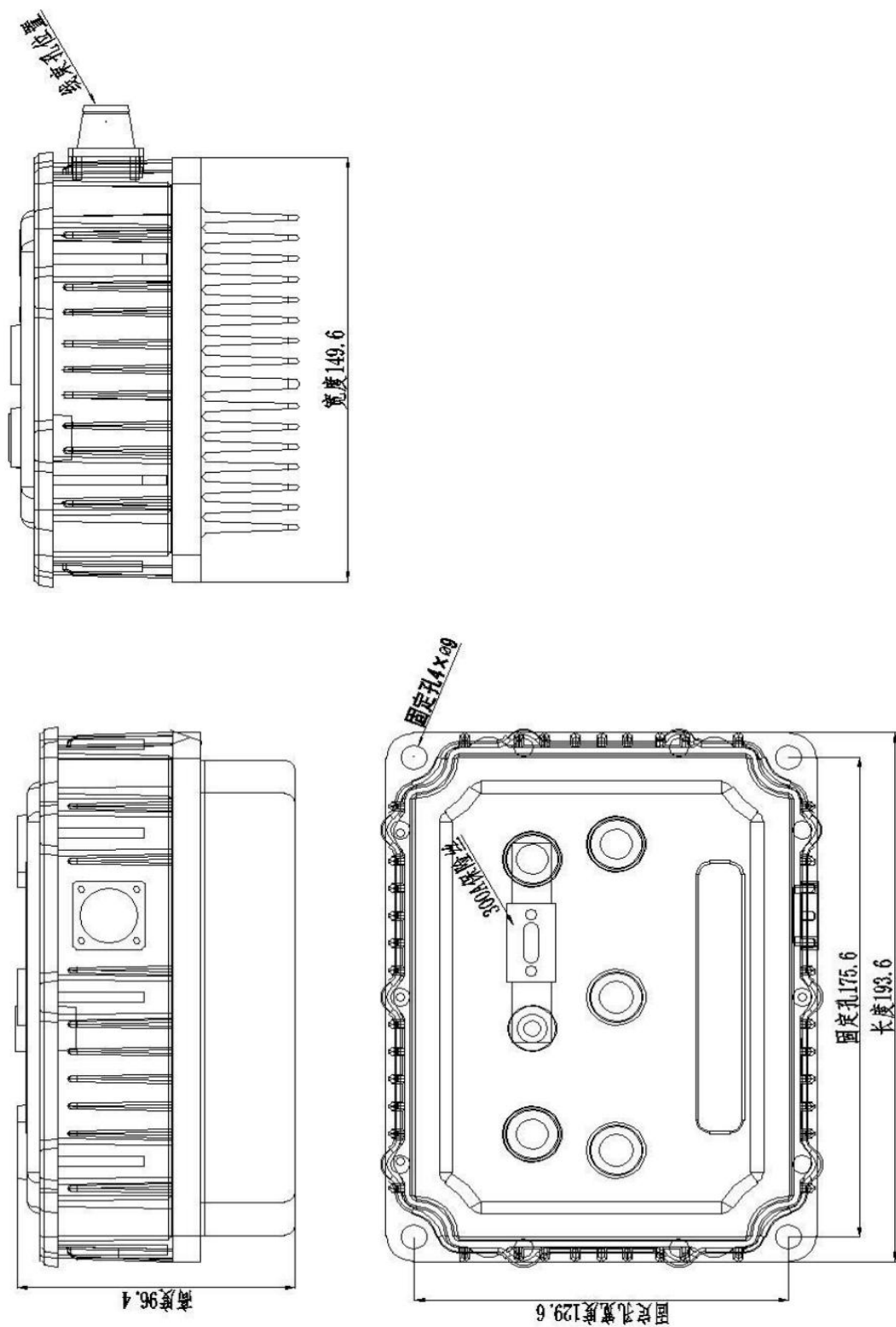
图一、5KW 控制器外形尺寸
